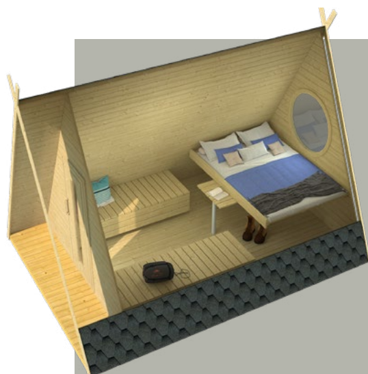
VOORBEELD Dwarsdoorsnede & inrichting
